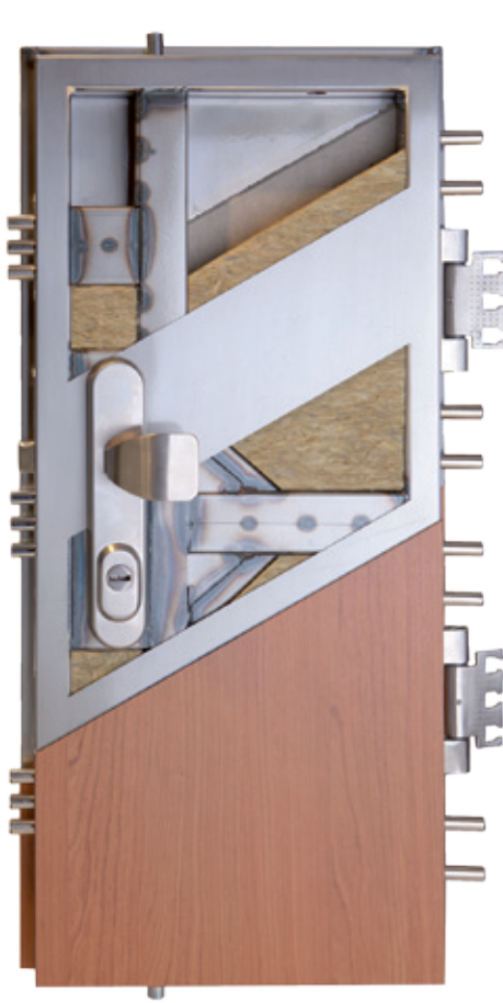
Řez dveří ŘADA ELITE
